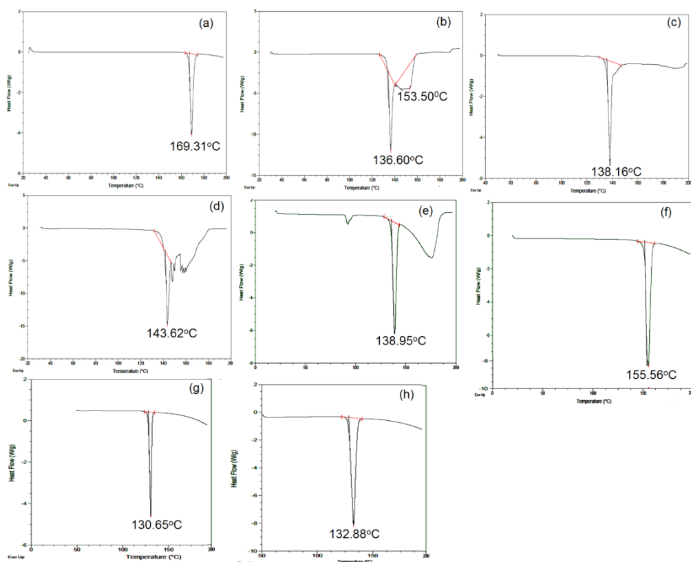
Figure S1. DSC thermograms of (a) LEF (b) SA (c) PA (d) MA (e) MOA (f) ADA (g) NA (h) INA.
